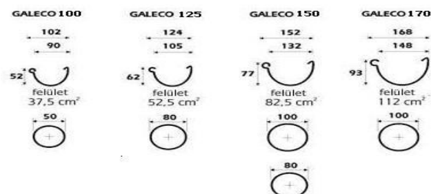
A Galeco PVC rendszerek átmérői
